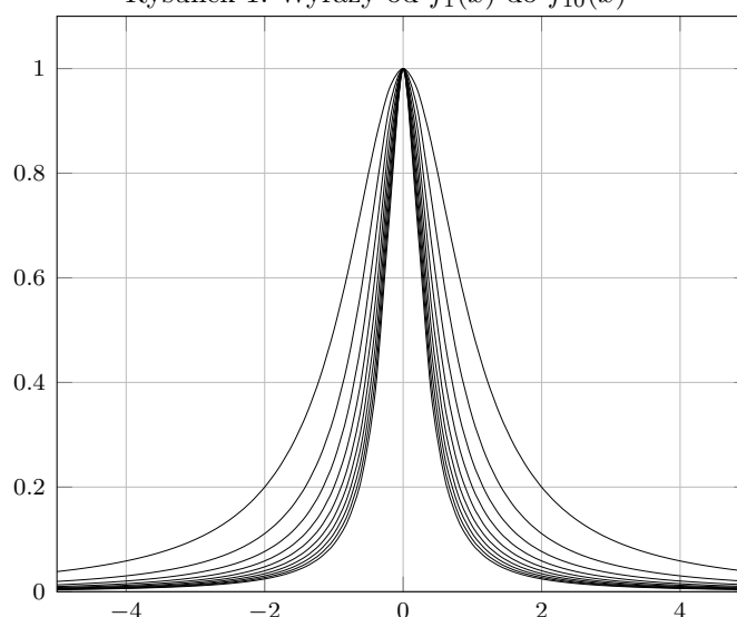
Rysunek 1: Wyrazy od f_1(x) do f_{10}(x)
